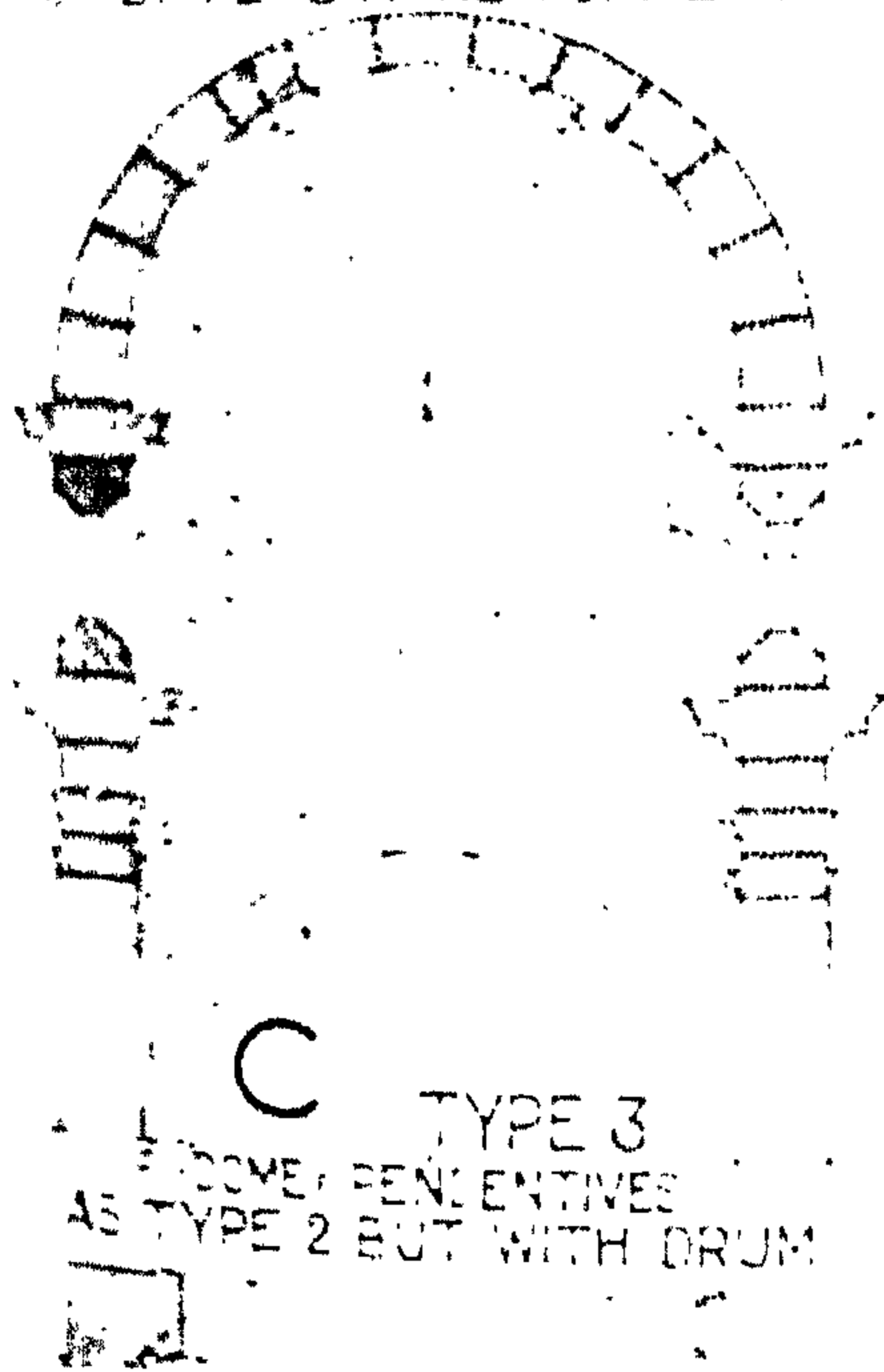
شكل (١٦) قباب مختلفة بأسلوب المعلقات (عن : Fletcher, p.603)
